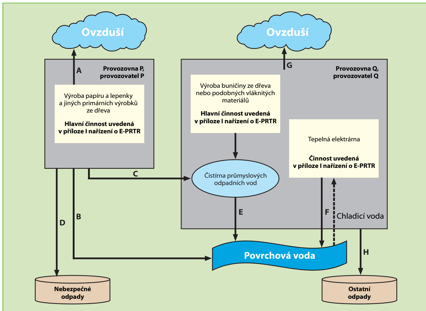
Obrázek 1: Průmyslový komplex se dvěma provozovnami s činnostmi podle přílohy I nařízení o E-PRTR
